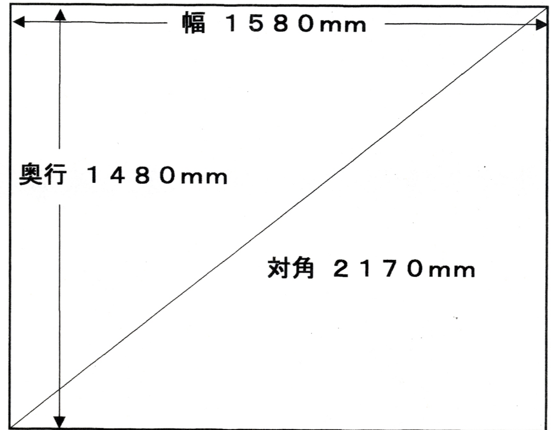
EV内扉寸法
